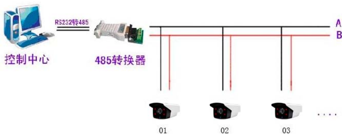
多个PTC052A 并联组网
